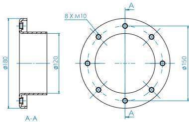
Flange (Ø180) size
